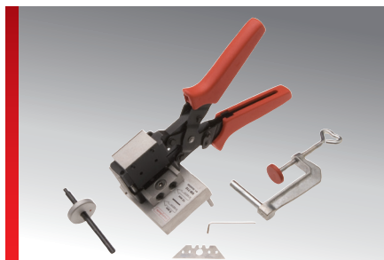
Комбинированный инструмент KM T10
